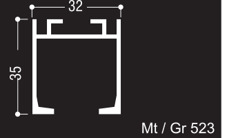
8019 - Üst Ray / Upper Rail
