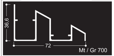
8025 - Üst Ray / Upper Rail
